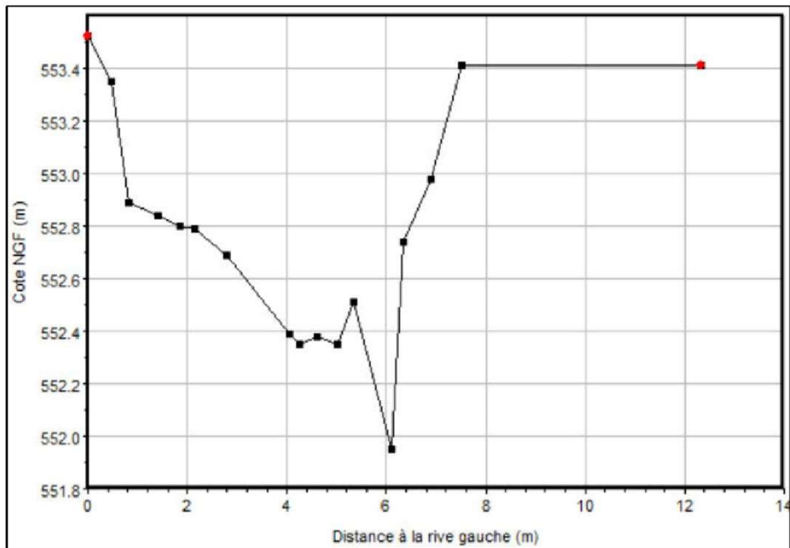
Figure 4 : Coupe de la brèche en rive gauche après restauration du barrage (vue depuis l'amont)
